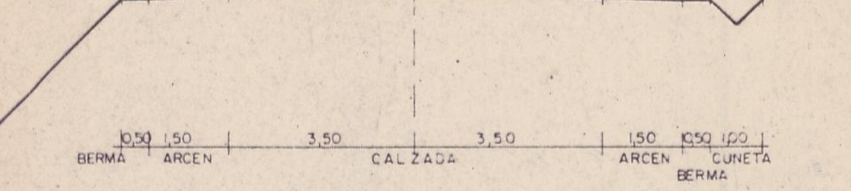
SECCION VIAL TIPO
