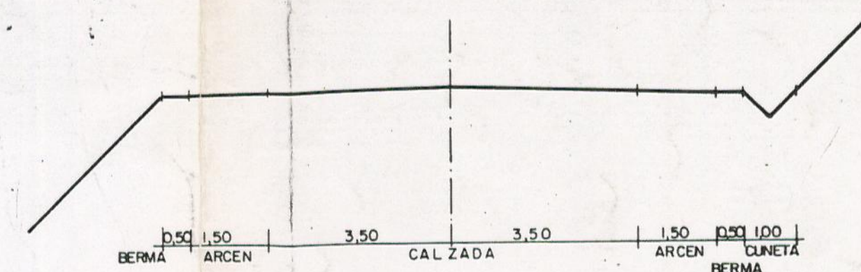
SECCION VIAL TIPO
