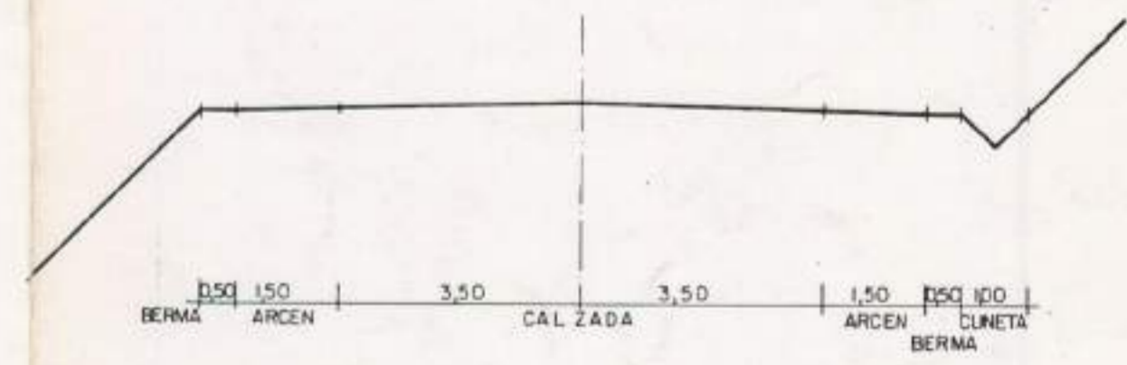
SECCION VIAL TIPO
