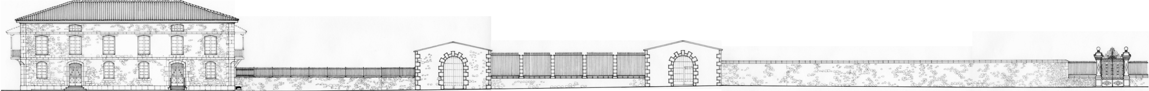
ALZADO C/ CAMILO ALONSO VEGA - PAR 1 de 3
